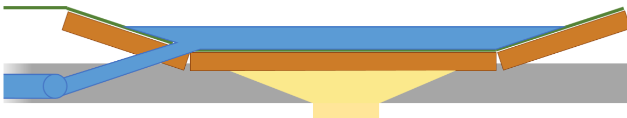
Figuur 6.4. Schematische weergave wadi (dwarsdoorsnede). In grijs de leemlaag, in blauw de vulling met water en de aansluiting op de riolering.
