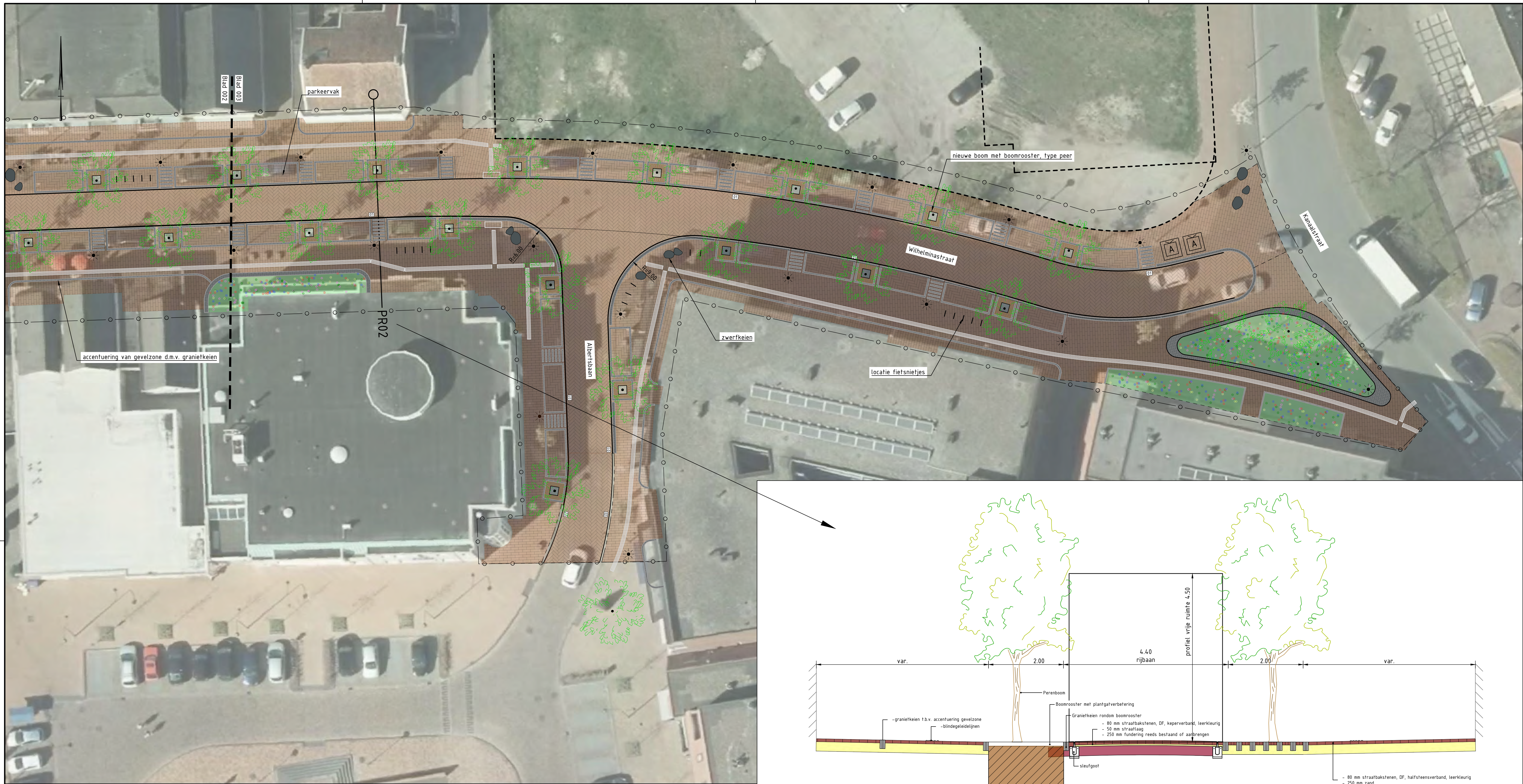
PR02 PRINCIEPPROFIEL WILHELMINAstraat schaal 1:50
