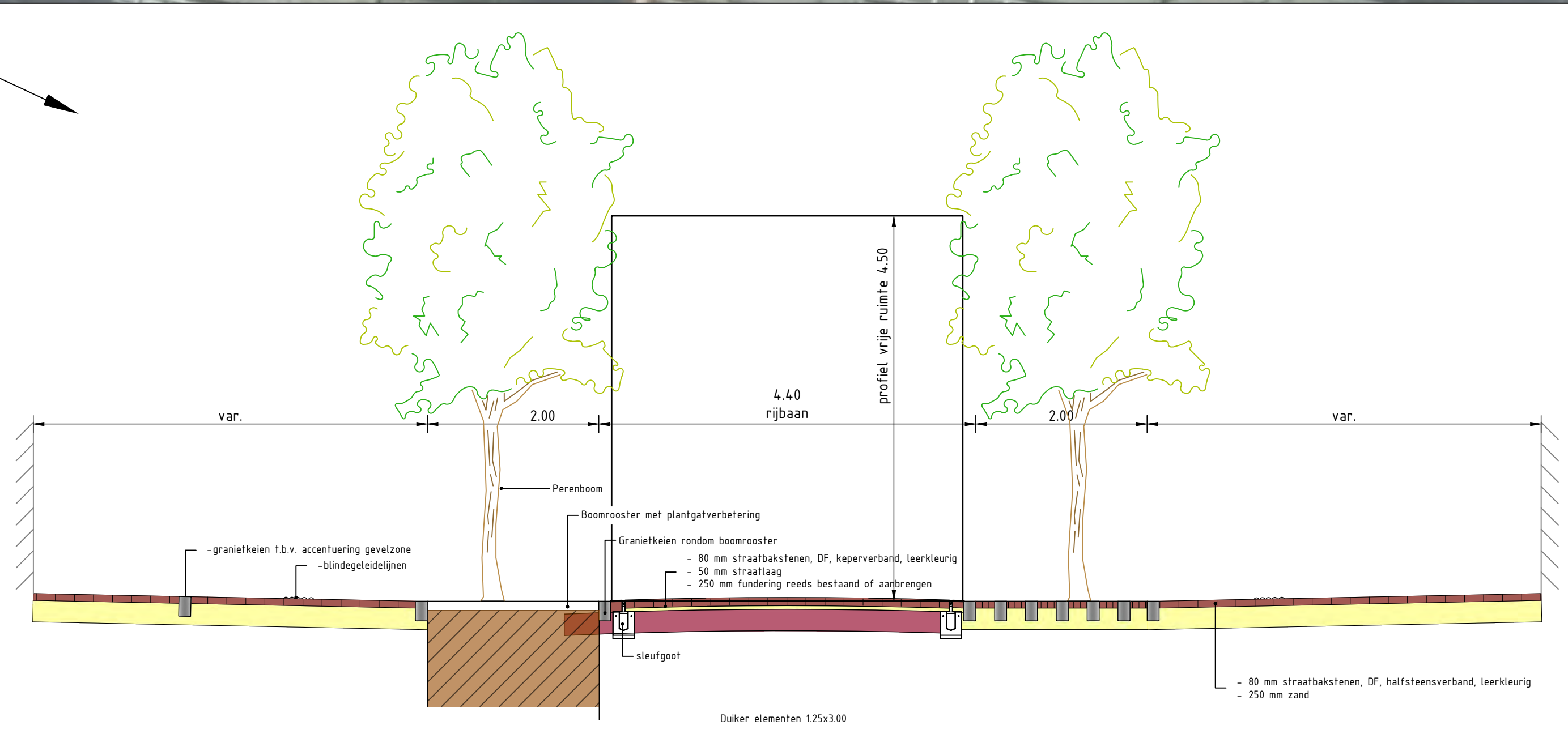
PR02 PRINCIEPPROFIEL WILHELMINAstraat schaal 1:50
